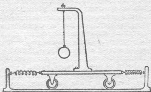
Рис. 1. Маятник на подвижной платформе
