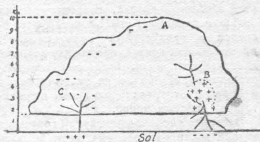
Рис 2 Образование грозового облака по Симсону
