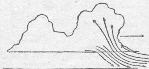
Рис. 1. Образование грозового облака
