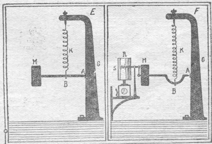
Рис. 3. E, F — вертикальные сейсмографы
